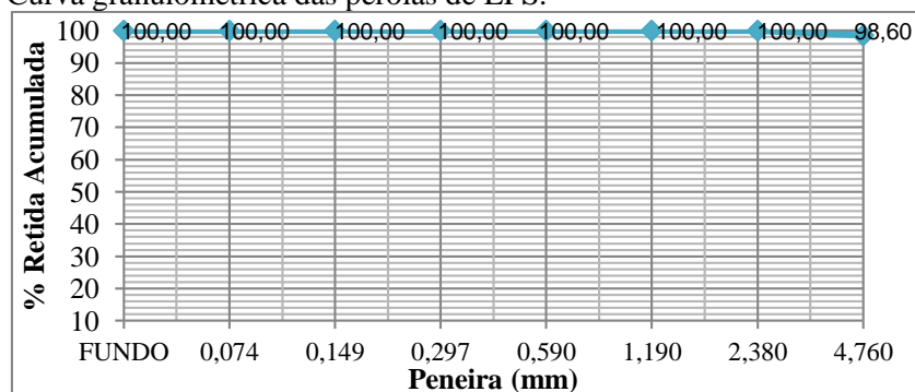
GRÁFICO 3 – Curva granulométrica das pérolas de EPS.
