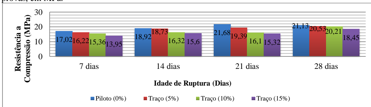
GRÁFICO 4 – Comparativo das Resistências Médias à Compressão nos diferentes traços de corpos de provas, em MPa.
