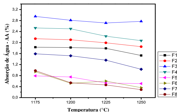
Figura 2. Ensaio de absorção de água (%) dos corpos-de-prova.
