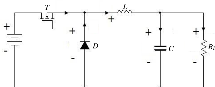
Figura 1. Circuito eletrônico do conversor Buck .
