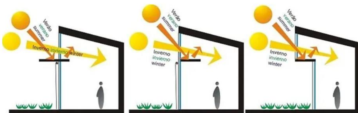
Figura 26. Formas de aproveitamento da luz natural em edificações com o uso de prateleiras de luz.
