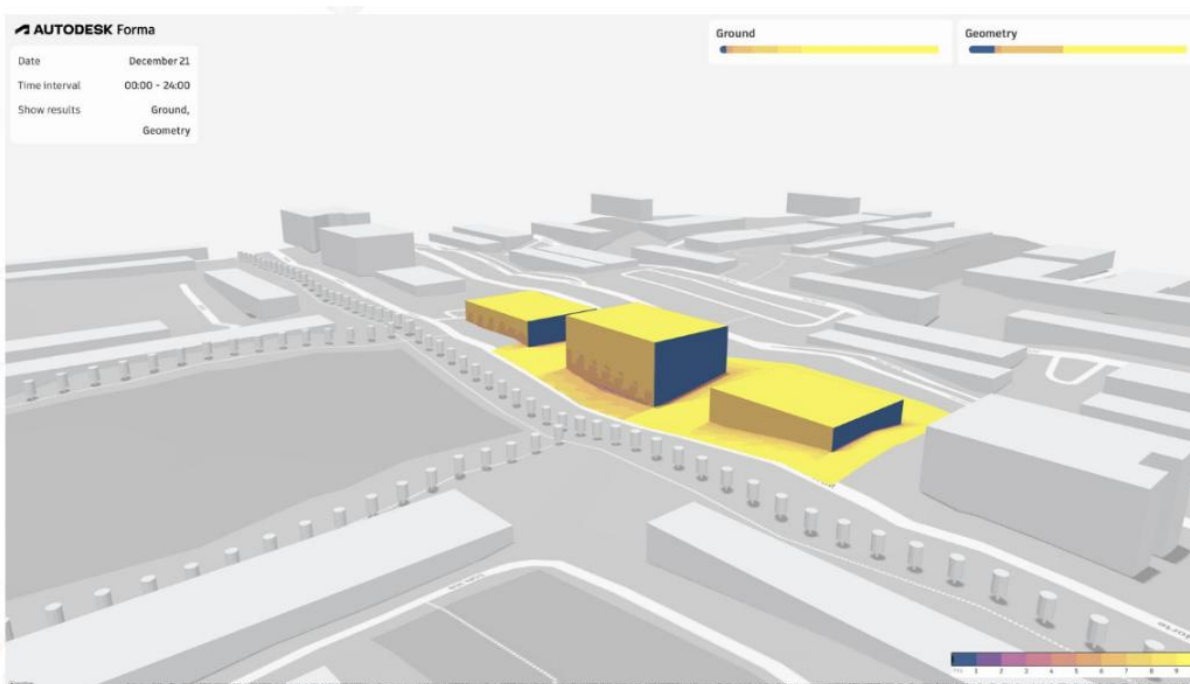
Figura 9. Incidência solar na face Noroeste em dezembro.
