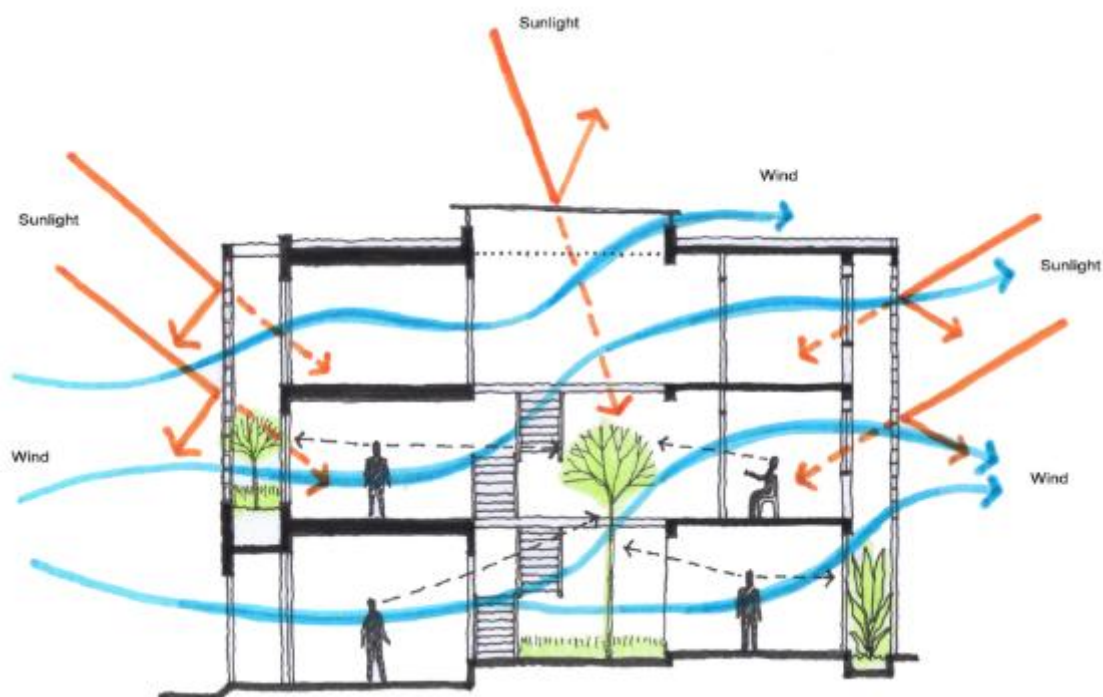
Figura 25. Estratégias de ventilação natural.
