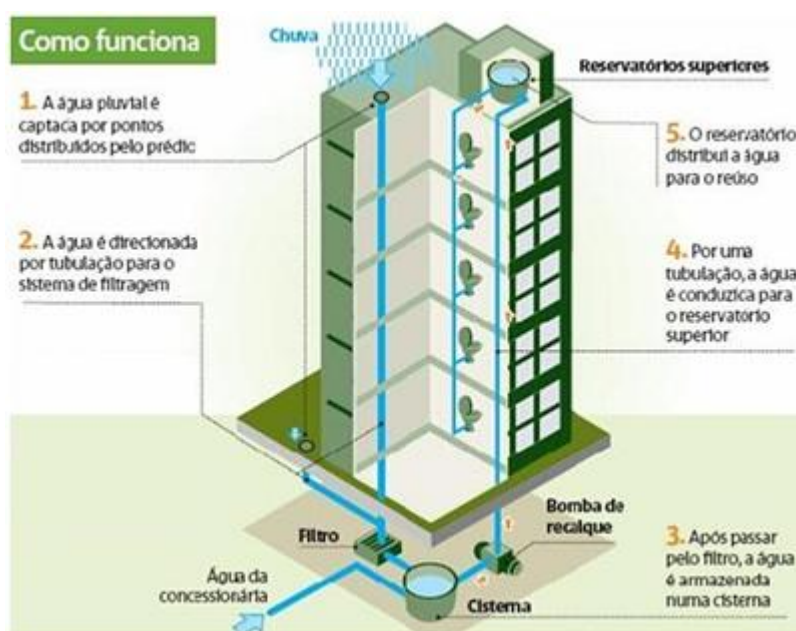
Figura 23. Sistema de captação de água da chuva para reaproveitamento.
