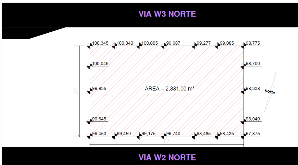
Figura 2. Terreno a ser considerado para a elaboração do projeto hachurado. Terreno com área de 2.331,00 m 2 . Fonte: Própria, 2025.
