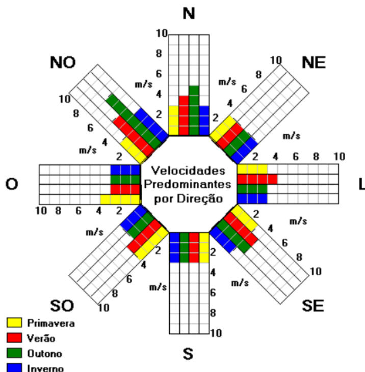
Figura 5. Gráfico de rosa dos ventos da cidade de Brasília/DF. Velocidades predominantes por direção.
