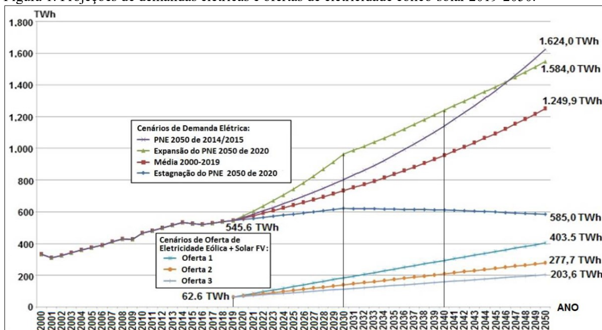
Figura 1. Projeções de demandas elétricas e ofertas de eletricidade eólico-solar 2019-2050.
