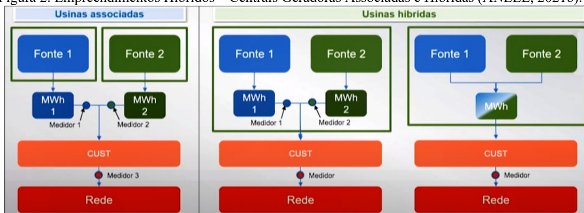
Figura 2. Empreendimentos Híbridos – Centrais Geradoras Associadas e Híbridas (ANEEL, 2021b).
