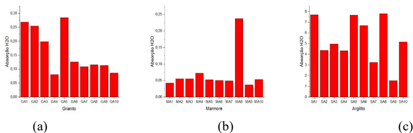
Figura 4 – Gráfico de absorção de água
