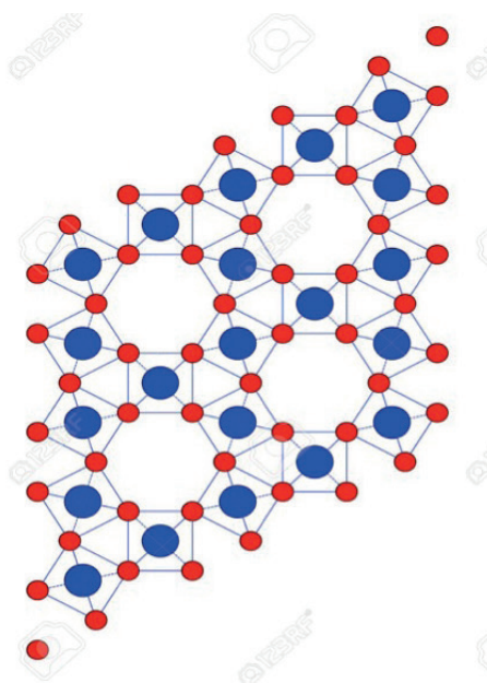
Figura 15 - Cristal de quartzo e sua estrutura cristalina - Oxigênio (Vermelho) e Silício (Azul)
