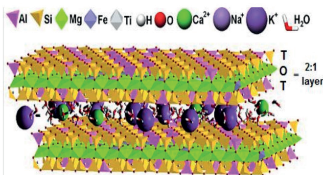
Estrutura cristaló-química de Vermiculita
