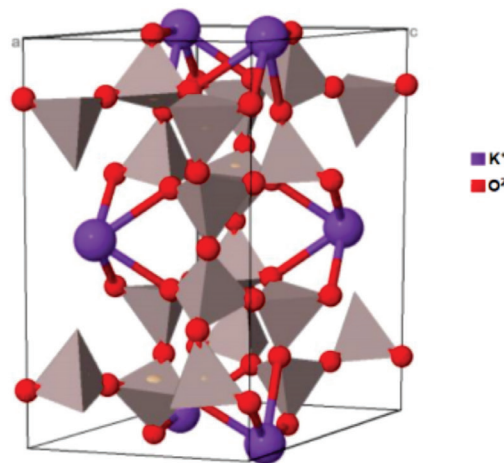
Figura 09 - Estrutura cristalina do mineral feldspato potássico
