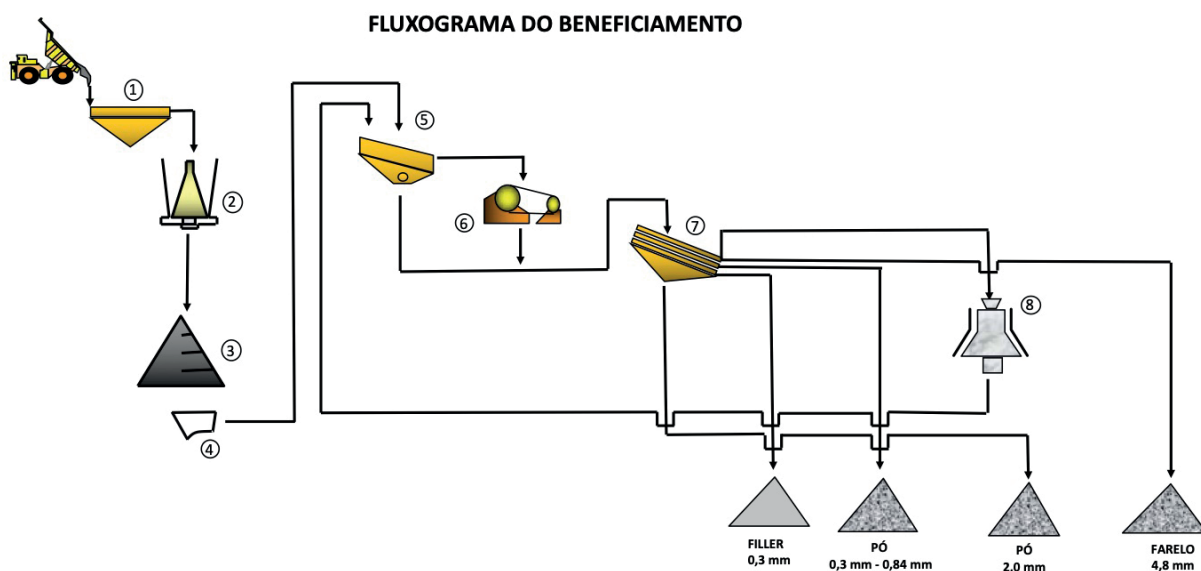
Figura 17 - Fluxograma esquemático do processo de beneficiamento dos remineralizadores
