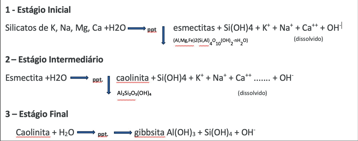
Figura 06 - Reações representando os estágios do Intemperismo em rochas silicáticas
