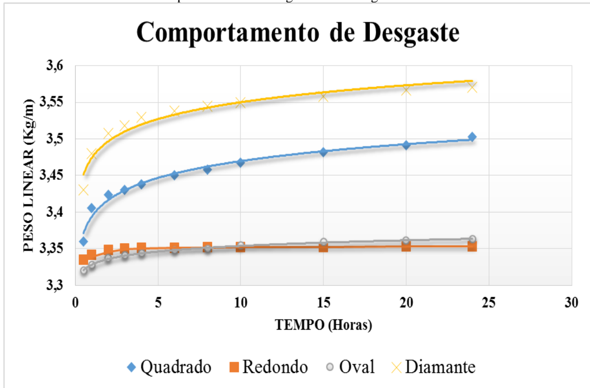
Gráfico 1. Tendência no Comportamento do Desgaste devido a geometria do canal.
